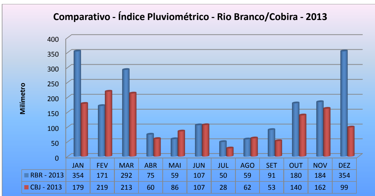
Gráfico 24 – Índice Pluviométrico (mm) – Rio Branco-AC/Brasil e Cobija – Pando/Bolívia - COMPARATIVO – ANUAL - 2013
