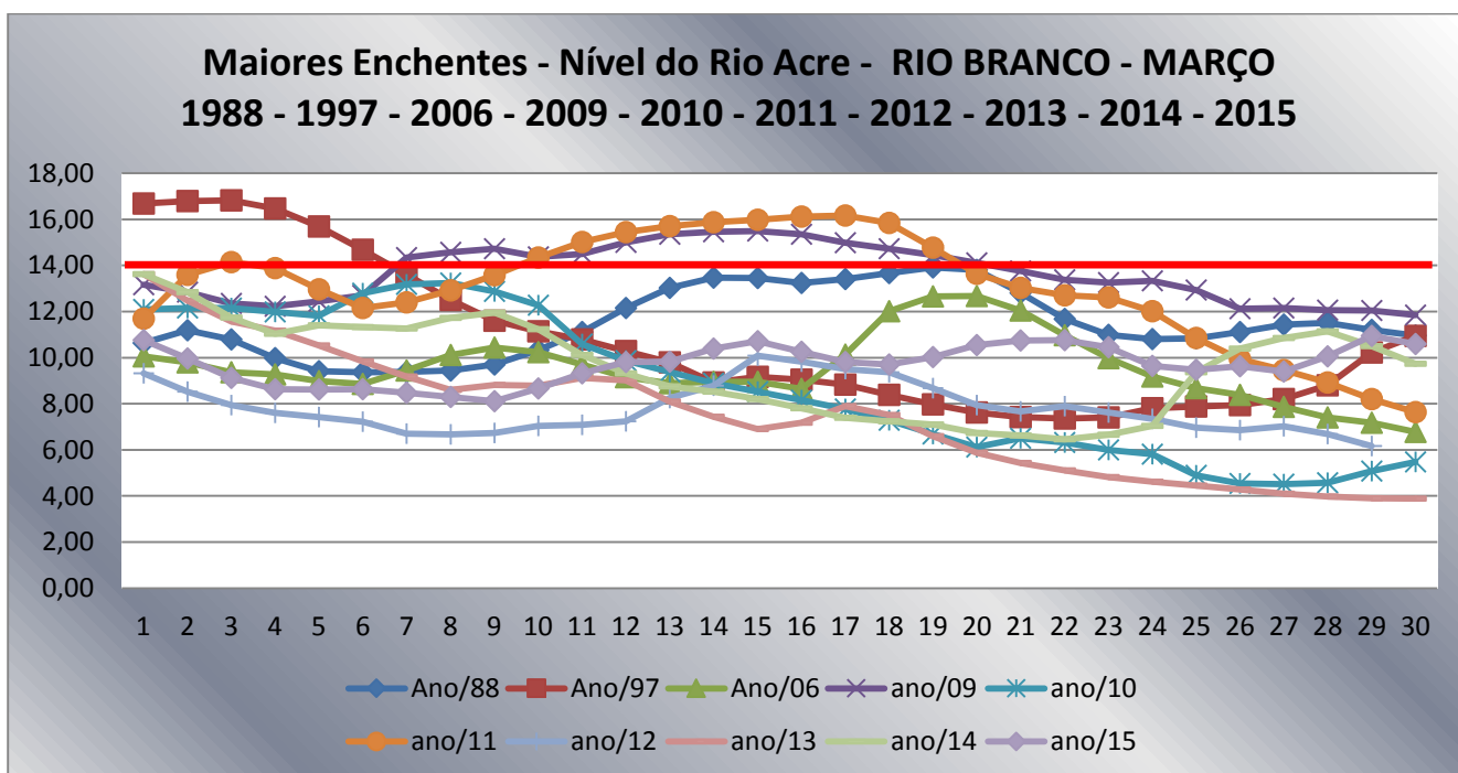
Gráfico 11 – Acompanhamento do Nível do Rio Acre (m), das Maiores Enchentes ocorridas. 1988-1997-2006-2009-2012-2011-2012-2013-2014-2015 Mês – ABRIL – RIO BRANCO
