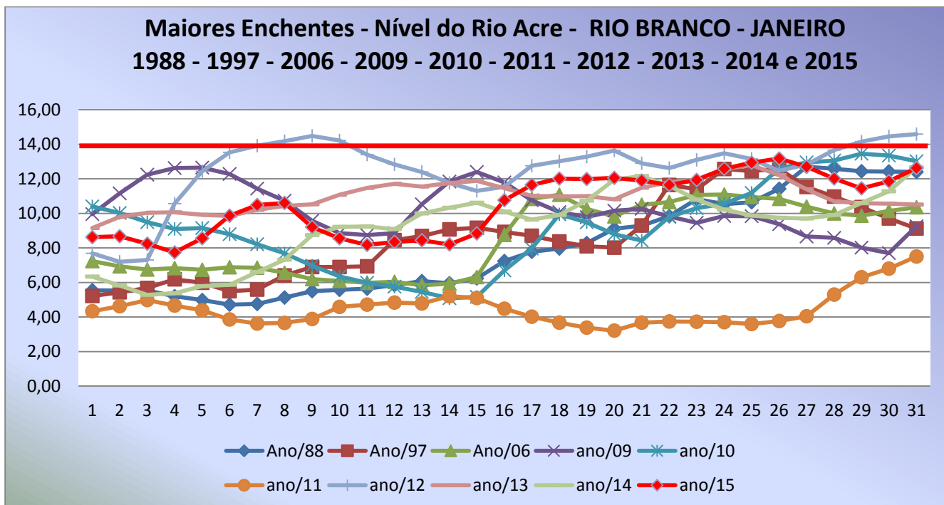
Gráfico 8 – Acompanhamento do Nível do Rio Acre (m), das Maiores Enchentes ocorridas. 1988-1997-2006-2009-2012-2011-2012-2013-2014-2015 - Mês – JANEIRO – RIO BRANCO
