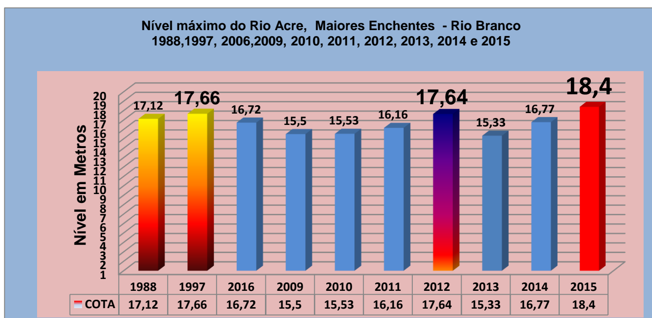
Gráfico 6 – Nível máximo do Rio Acre (m), em Rio Branco Maiores Enchentes de 1988, 1997, 2006, 2009, 2010, 2011, 2012, 2013, 2014 e 2015
