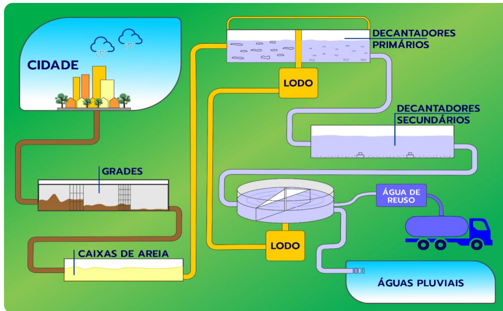
Figura 16 – Modelo de drenagem urbana e reuso de águas pluviais
