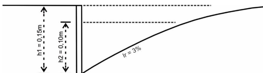
Figura 26 – Declividade da rua e altura da água na sarjeta
